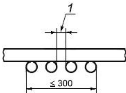
Рисунок 1 - Кабели, закрепленные на передней стороне стандартной лестницы с зазором
