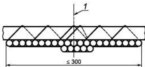
Рисунок 3 - Кабели, закрепленные на передней стороне стандартной лестницы без зазора (комплекты отрезков кабелей находятся в контакте)
