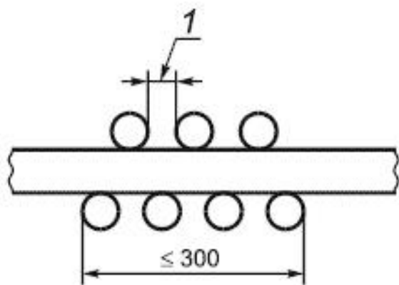
Рисунок 1 - Типичное расположение с зазором кабелей, закрепленных на обеих сторонах стандартной лестницы (категория A F/R)
