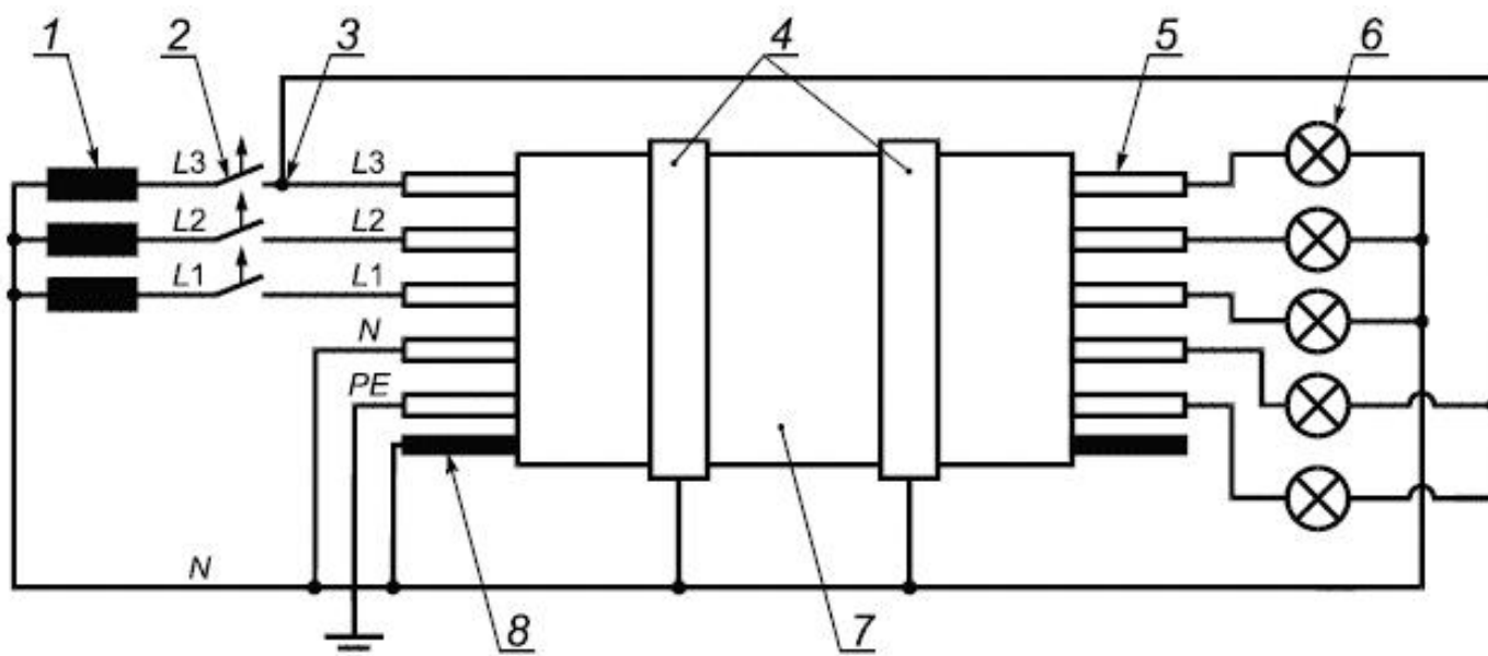
Рисунок 3 - Схема основных соединений
