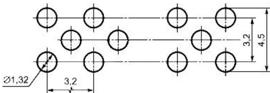
Рисунок 5 - Фронтальная поверхность горелки
