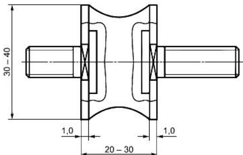
Рисунок 4 - Типовая резиновая втулка для крепления испытательной лестницы
