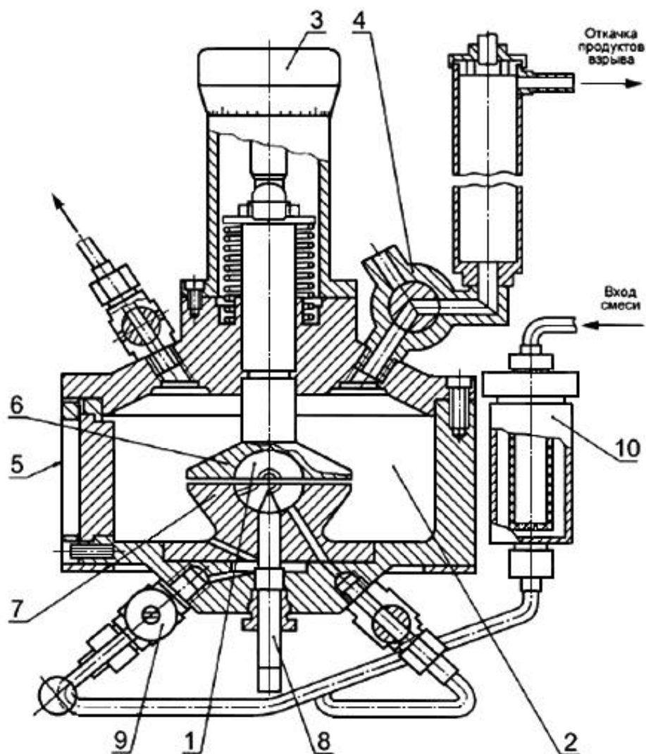
Рисунок 1 - Установка для определения БЭМЗ
