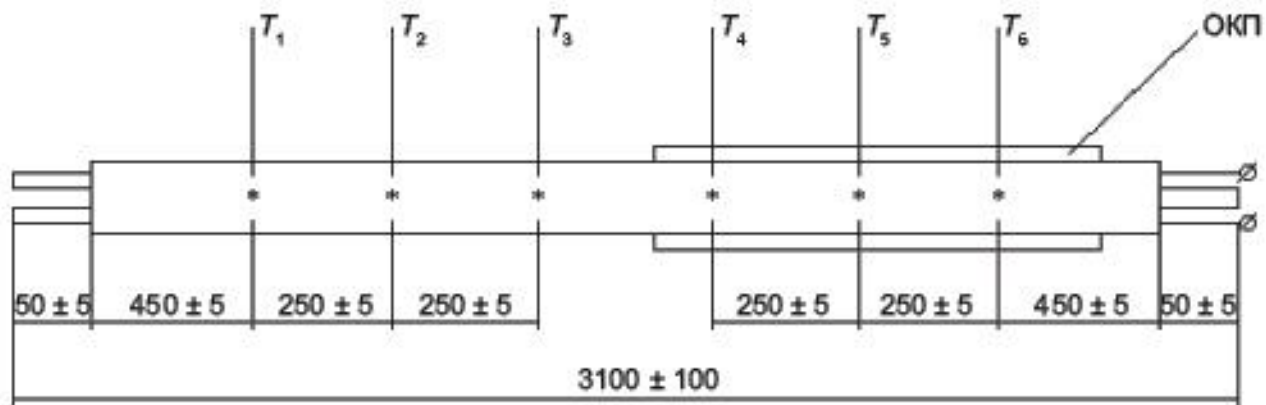
Рис.1 - Размещение термоэлектрических преобразователей
