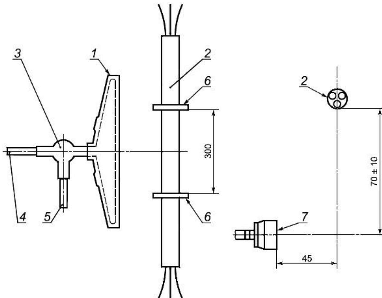
Рисунок 4 - Расположение горелки и образца кабеля при испытании
