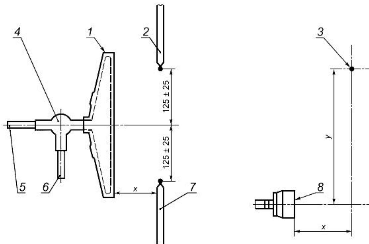
Рисунок А.1 - Расположение термодпар при проверке
