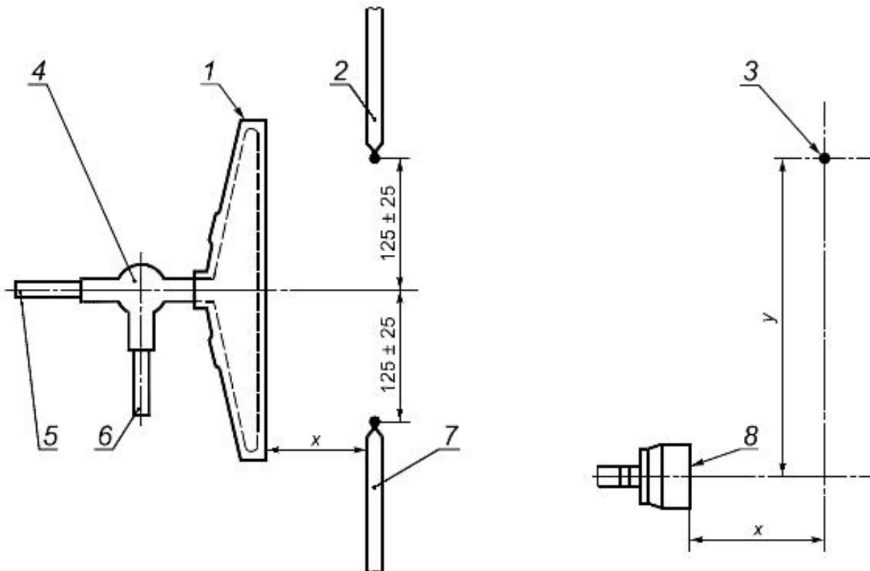
Рисунок А.1 - Расположение термодпар при проверке
