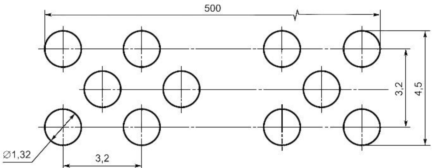
Рисунок 2 - Фронтальная поверхность рабочей части горелки
