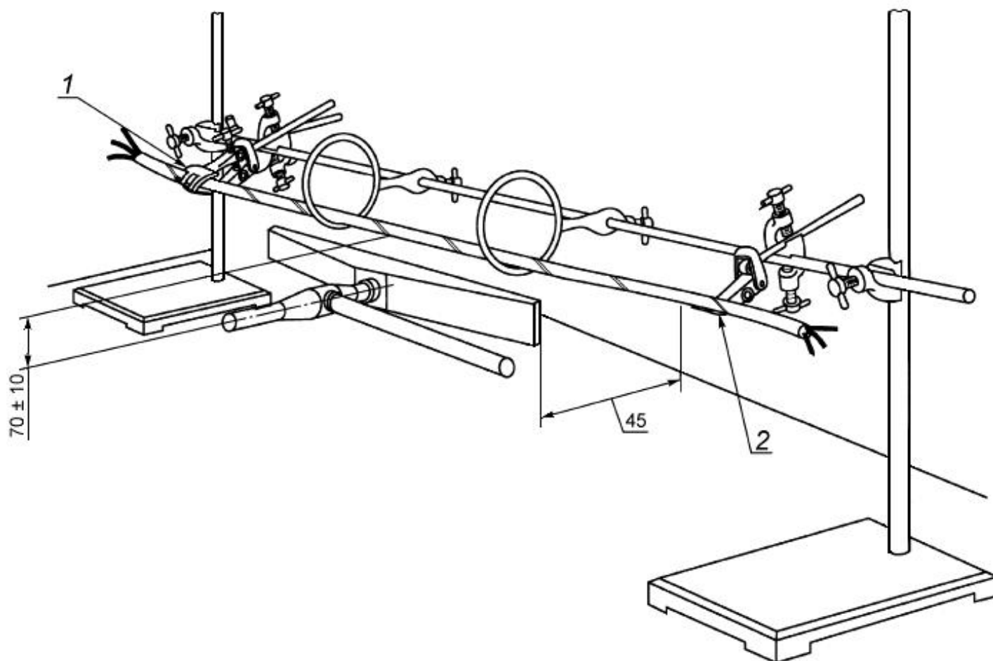
Рисунок 1 - Пример поддерживающего устройства
