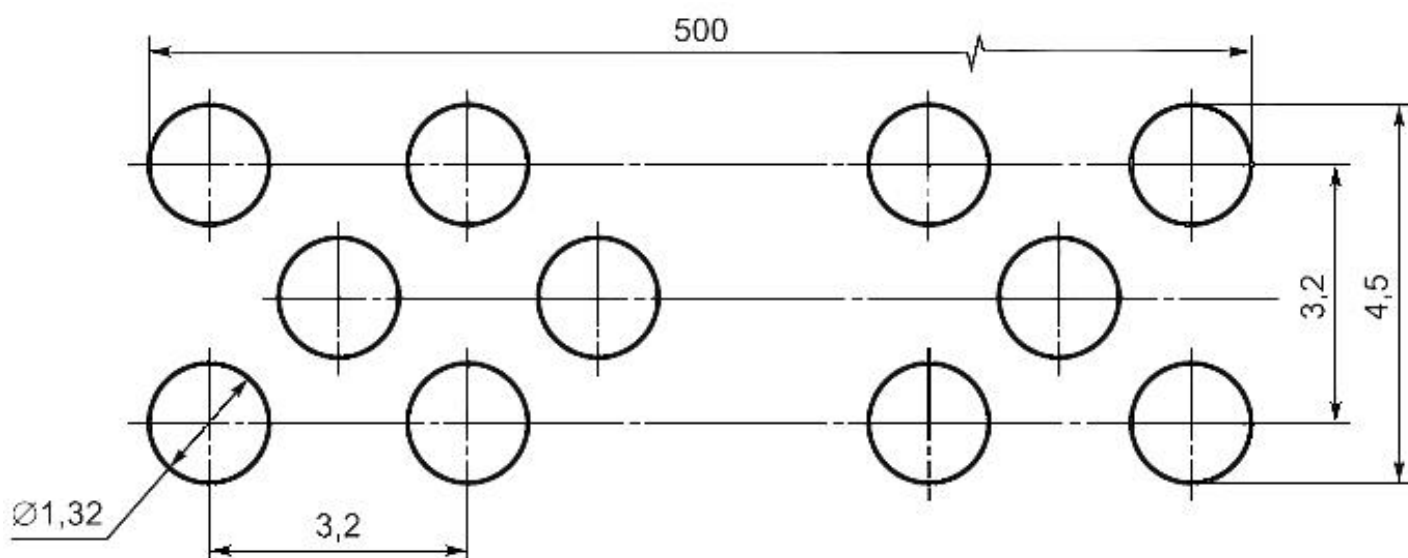
Рисунок 2 - Фронтальная поверхность рабочей части горелки
