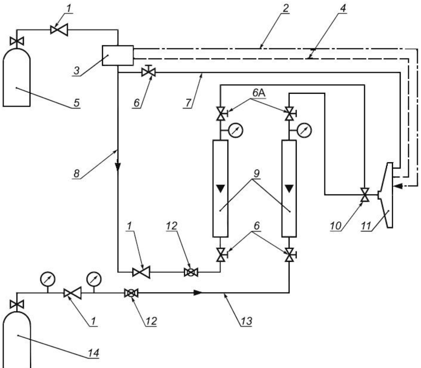
Рисунок 3 - Примерная схема системы контроля работы горелки с использованием ротаметров
